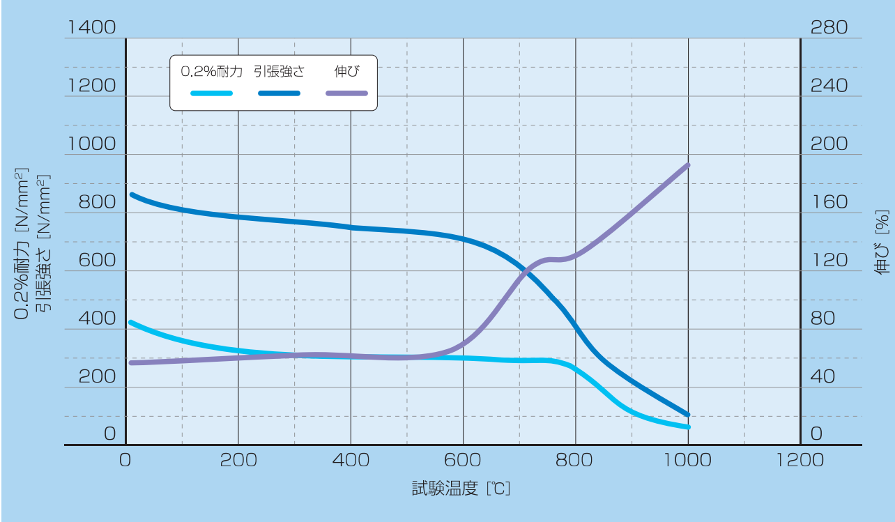
高温引張試験結果 (焼なまし材)
