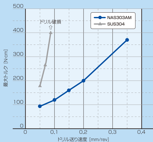
NAS303AMとSUS304の切削抵抗テスト結果 板厚10mm、ドリル回転数1,500rpm
